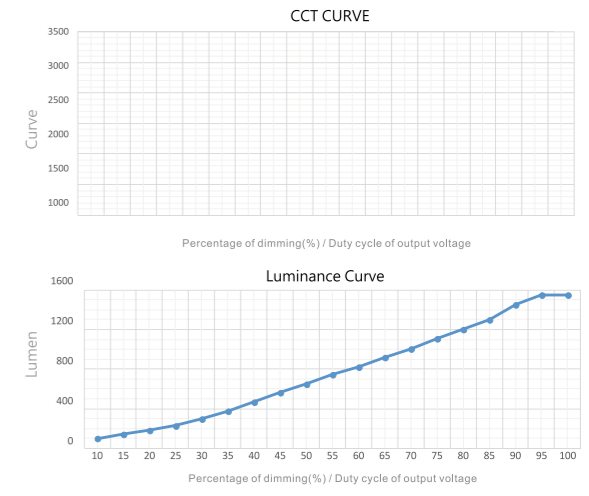
調光曲線 (Base on Ip20 CRI > 90)
